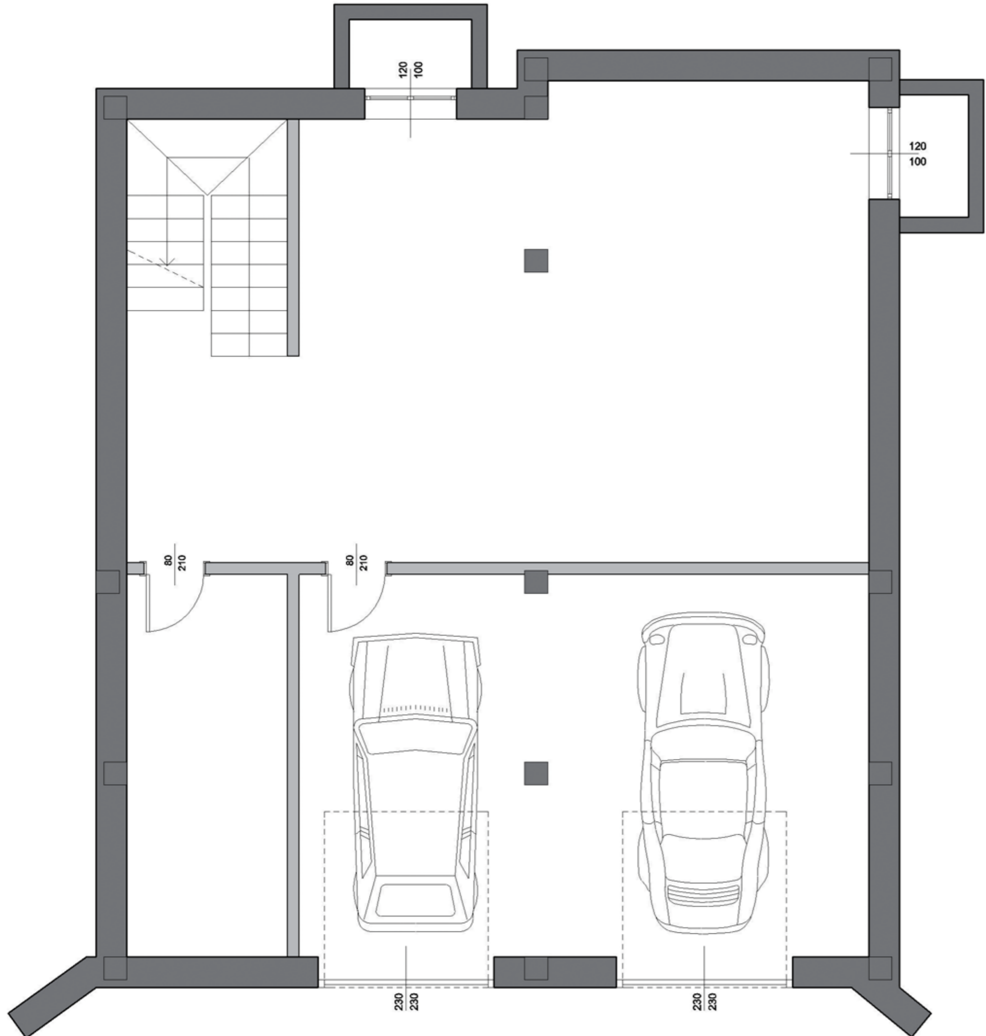
VILLA SINGOLA "A" PIANO INTERRATO sup. commerciale mq. 125.87
