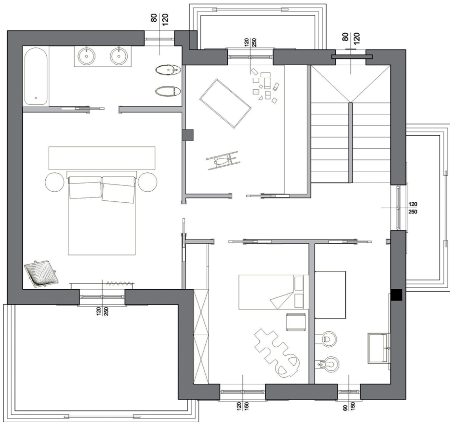
VILLA SINGOLA "A" PIANO PRIMO sup. commerciale mq. 87.85 sup. balconi mq. 22.02
