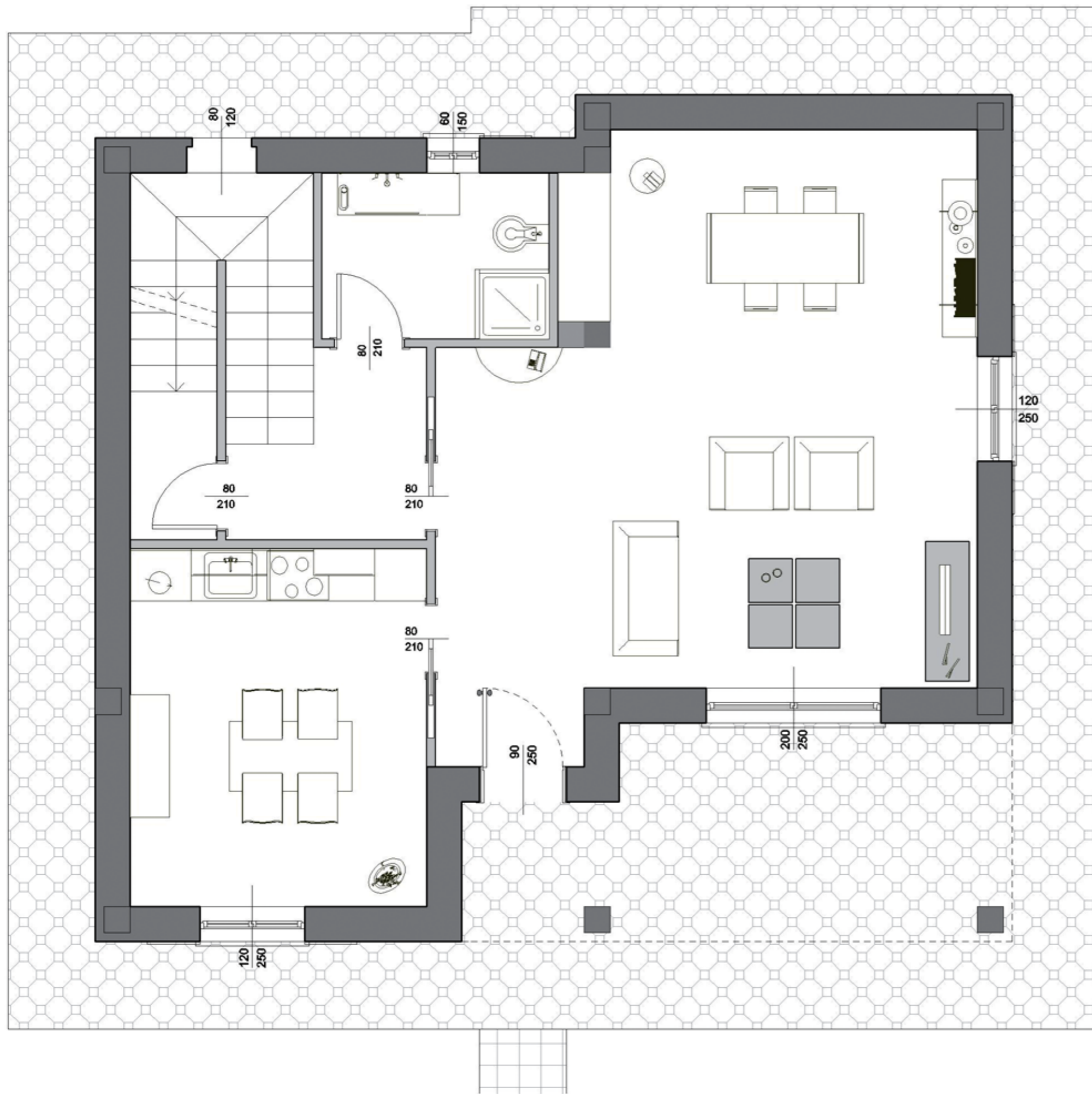
VILLA SINGOLA "A" PIANO TERRA sup. commerciale mq. 84.98 sup. portico mq. 14.13
